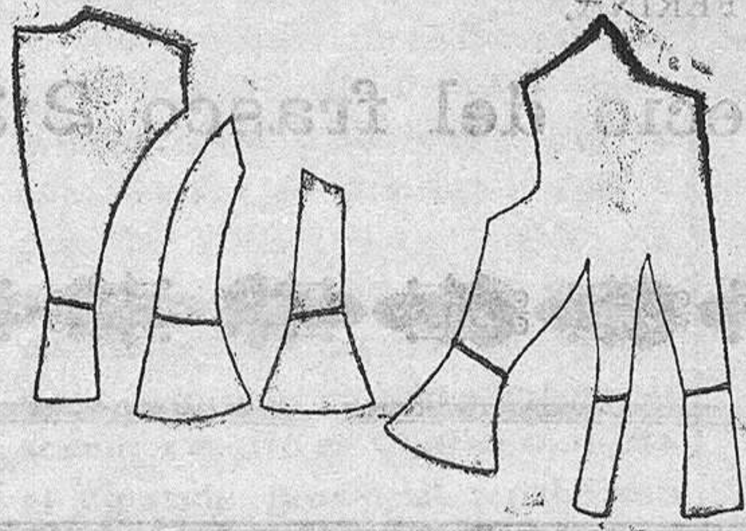
23-24 m. y
