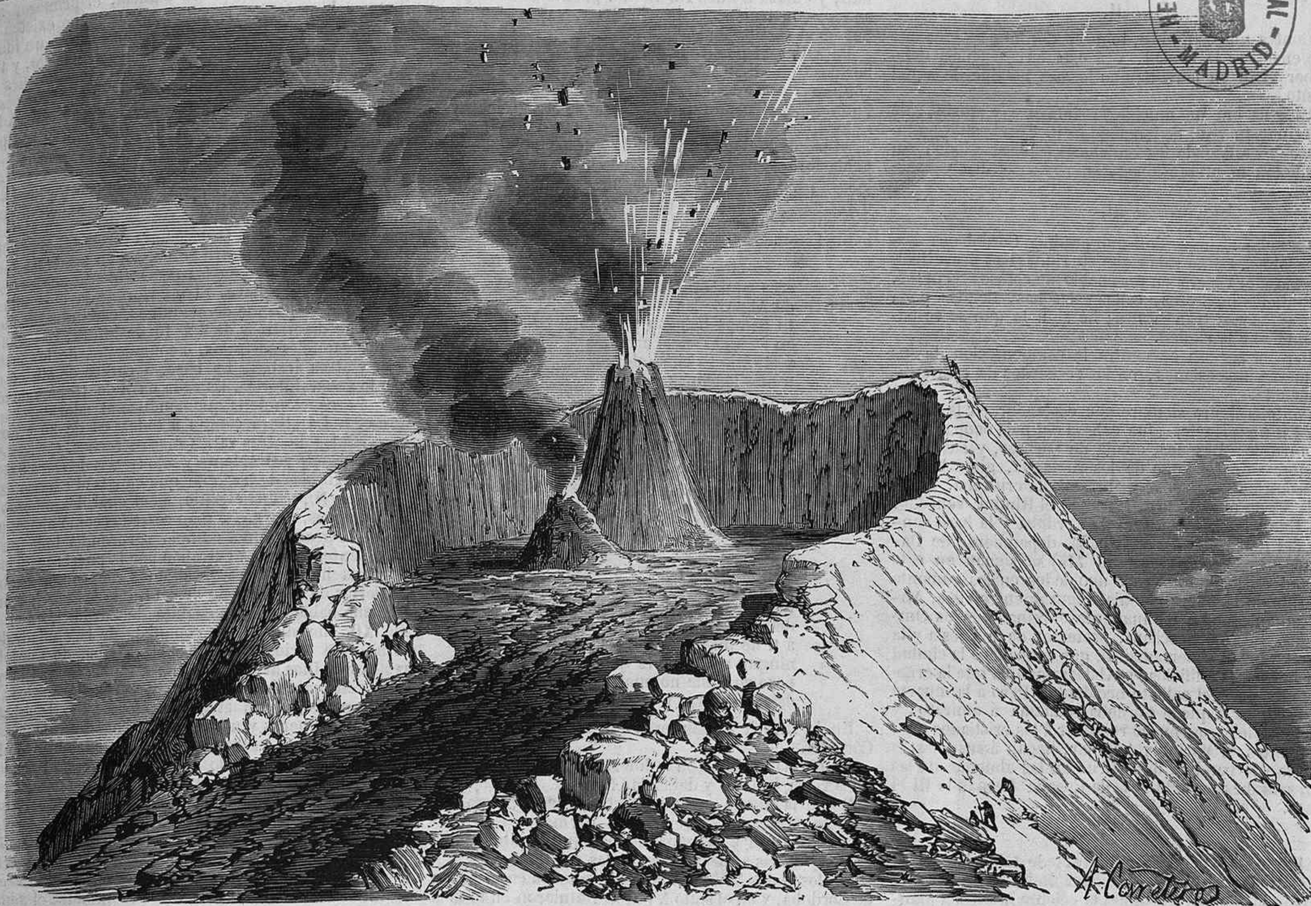
ITALIA. — VISTA DE LA ÚLTIMA ERUPCIÓN DEL VESUBIO.
