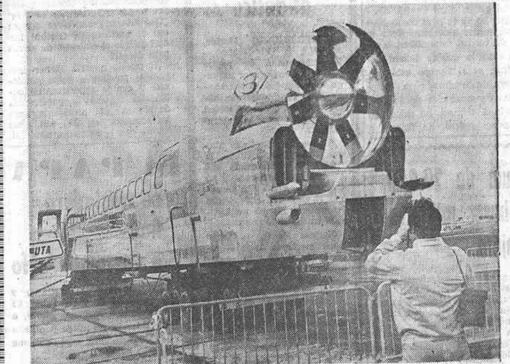
PARIS. — La parte trasera del primer aerotrén operacional, mostrado a la prensa en el aeropuerto de Le Bourget. La propulsión se realiza por dos turbo motores "Turmo III E 3", de 1.300 H.P. cada uno
