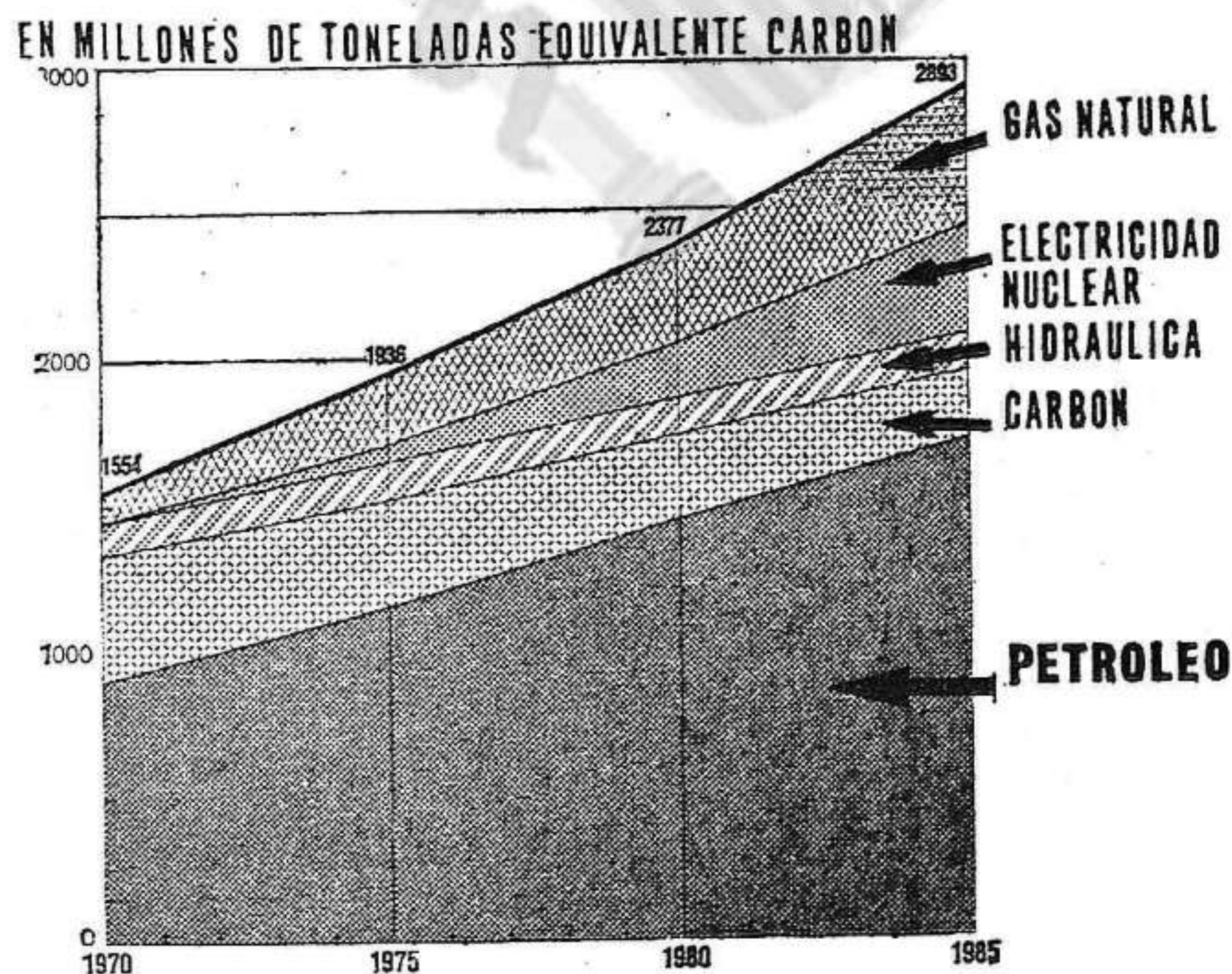
Previsiones del consumo de energía en Europa Occidental
