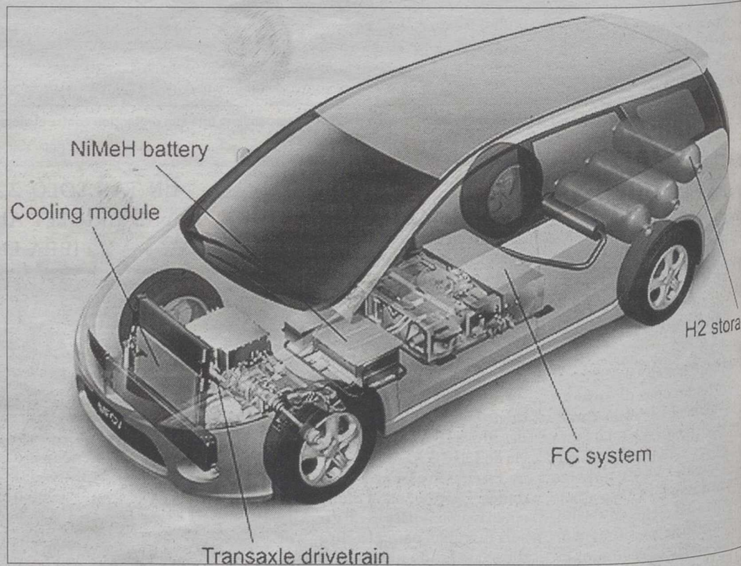
Esquema de la célula de combustible desarrollada para el Mitsubishi Grandis.
