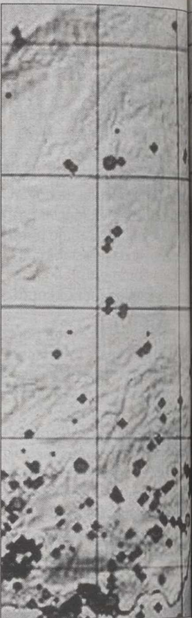
Seísmos registrados en 2000. / ICA
