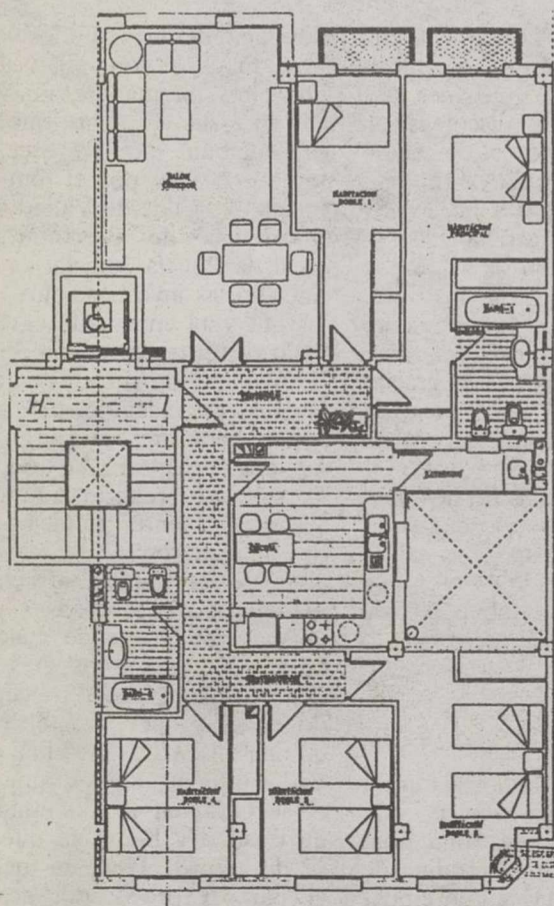
VIVIENDA TIPO I.
