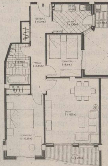
Vivienda tipo "B" Superficie útil=64,65m 2 (planta 1)
