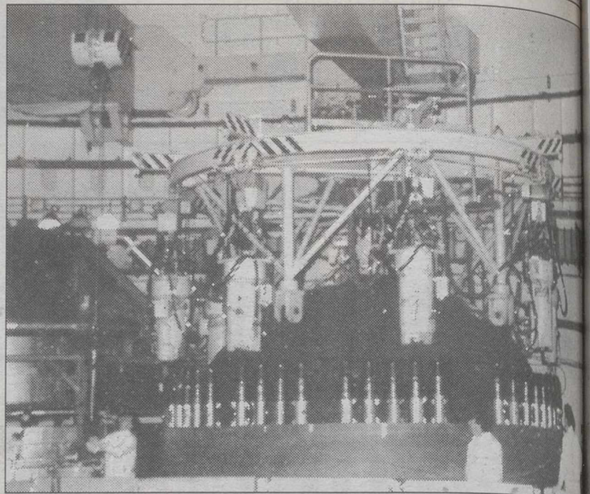
Tapa de la vasija del reactor de la nuclear de Cofrentes.
