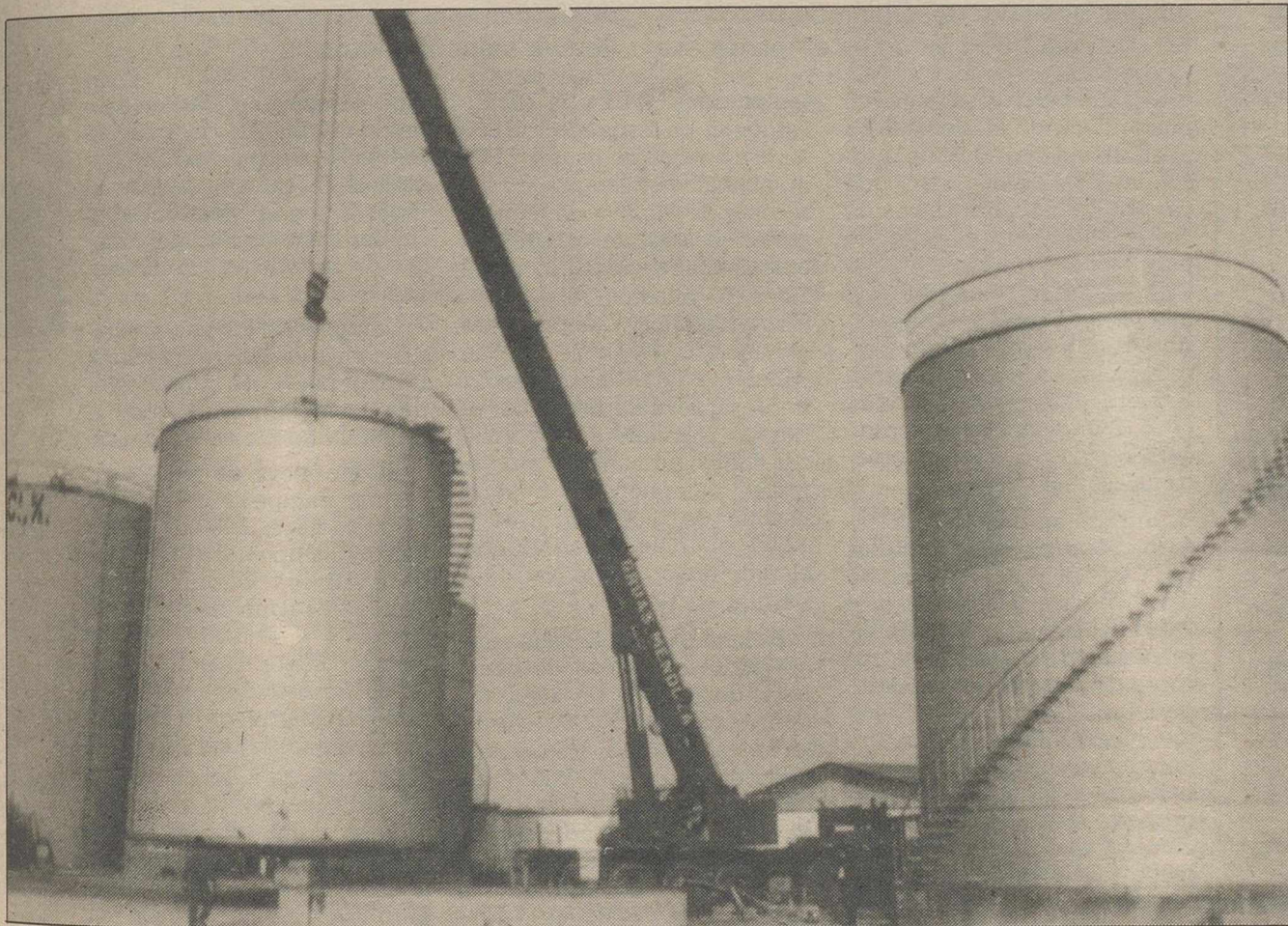
Depósitos de acero inoxidable para vinos, mostos, leche y, en general, para la industria alimentaria
