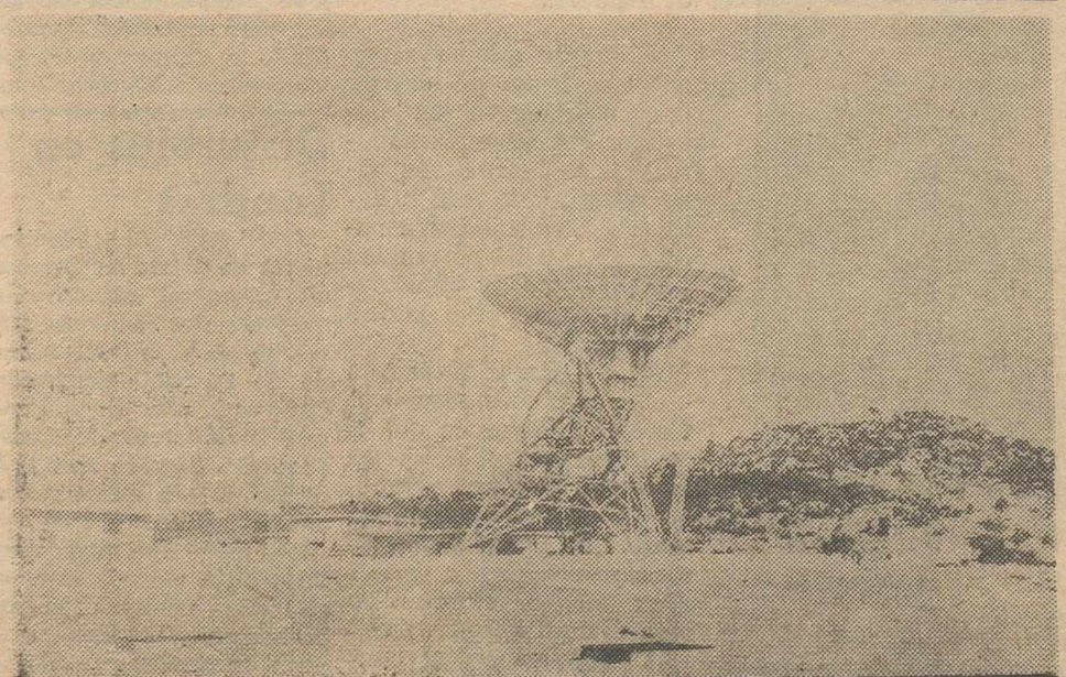
Esta es la gran antena parabólica de 26 metros de diámetro y 250 toneladas de peso de la Estación Espacial de Robledo de Chavela, con la que se recibirán las señales del "Lunar Orbiter" y las fotografías que transmite. Se anuncia que la recepción en Robledo de las fotografías será el 19 de agosto. (Foto EUROPA PRESS)
