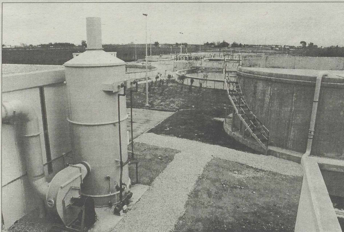
Nueva planta de tratamiento del agua en Manzanares.
