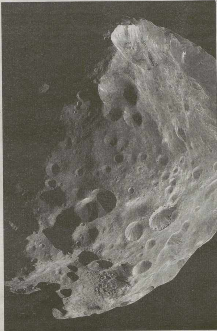
Un fósil cósmico. Febe, la luna negra de Saturno, es un fósil congelado que nació en los primeros momentos del Universo, hace cuatro mil millones de años, según los datos transmitidos a Tierra por la sonda espacial Cassini-Huygens, y que desveló ayer la NASA. / FOTO: AP
