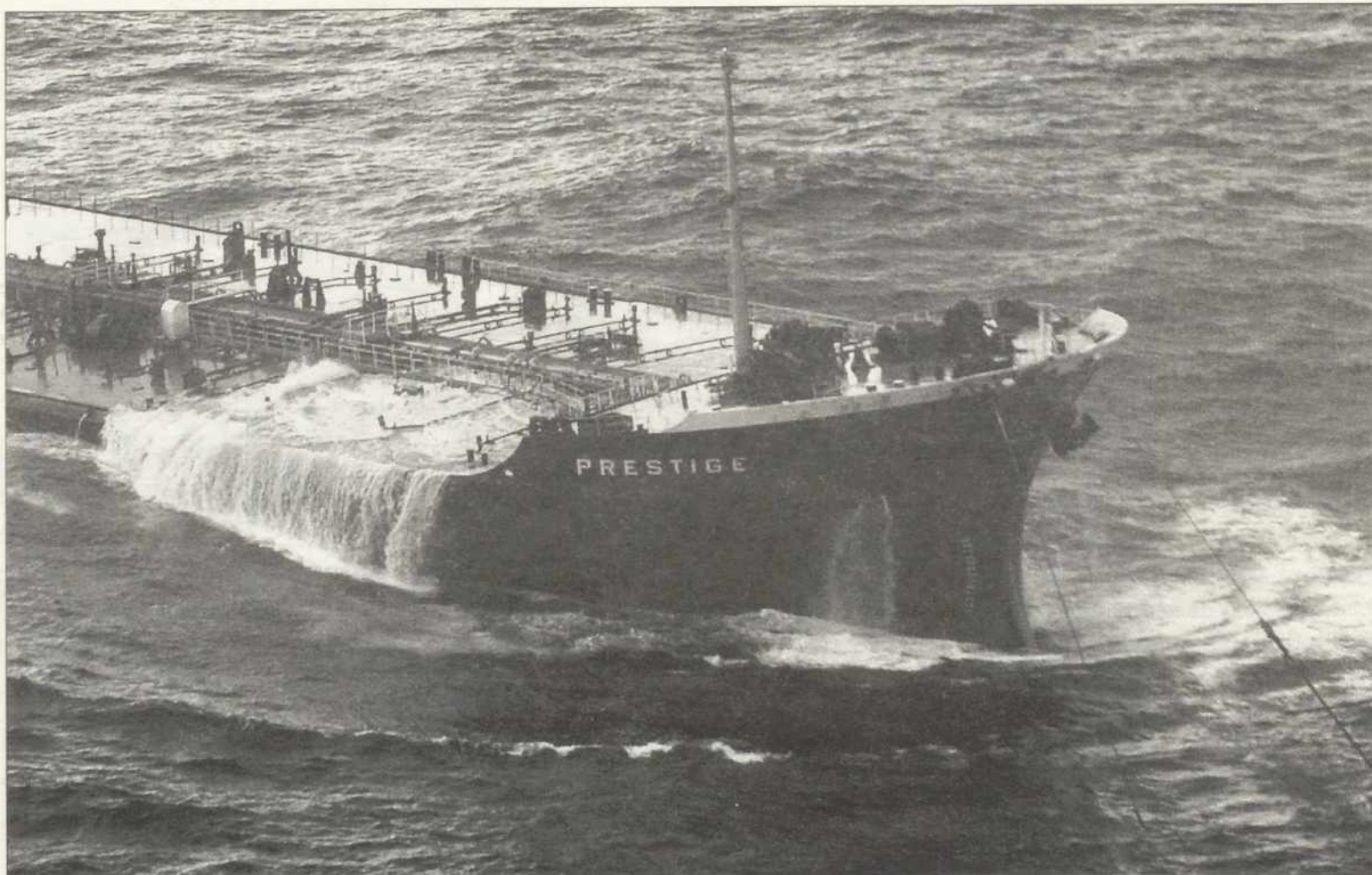
El petrolero 'Prestige' echa agua al mar después de que Salvamento Marítimo lograra enderezarlo y evitar su hundimiento frente a las costas gallegas. / EFE
