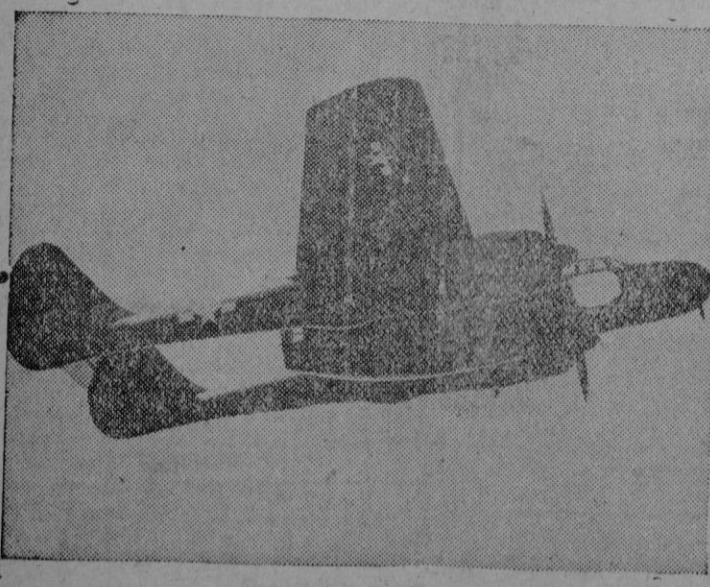
El nuevo avión norteamericano "Black Widow", primer caza nocturno de la guerra, realizando un vuelo de prueba en los EE. UU.
