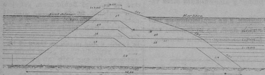
(Fig. 14) — Perfil del dique principal del Nuevo Puerto
