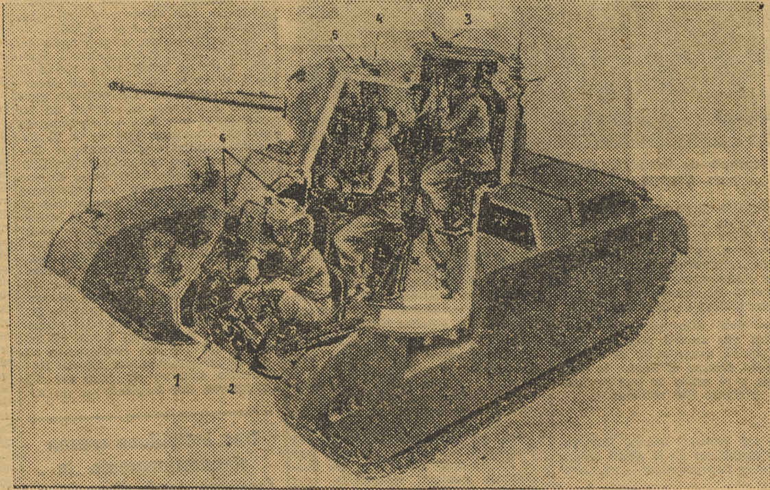
Los tanquistas mantienen secretos, en lo posible, los detalles de sus tanques. Este croquis no representa un tipo determinado. Da tan solo la posición general de los tripulantes de un tanque moderno:
