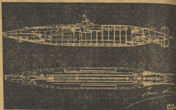
Planos del submarino de Isaac Peral, dibujados por el mismo inventor, cuya firma reproduce el grabado (Fotos Cifra)
