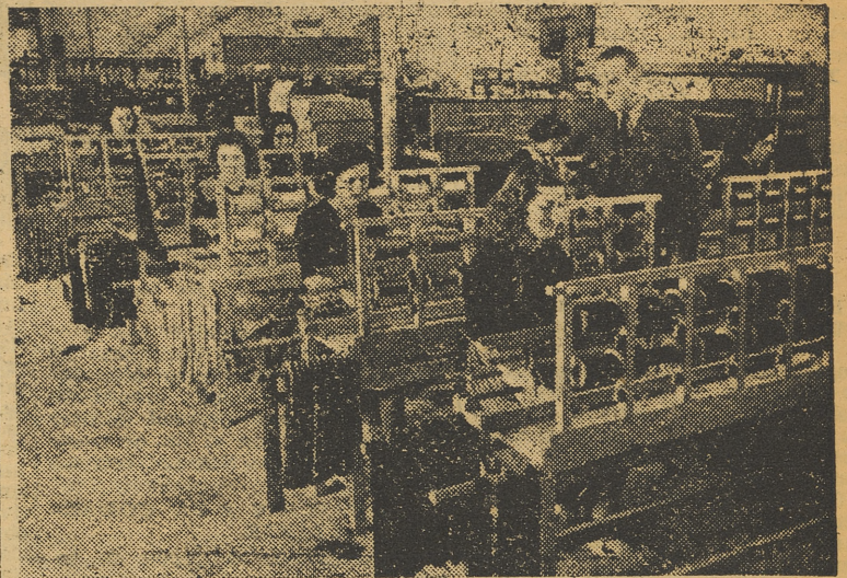
Preparación de las bobinas o carretes de hilo de seda
