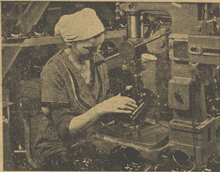
Fabricación de cajas de teléfono de material comprimido. con una fresa se elimina la rebaba que se forma en el prensado
