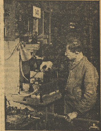
Fabricación de piezas de material comprimido.— La masa suministrada en forma de tabletas para facilitar la carga, se introduce en el molde de prensado
