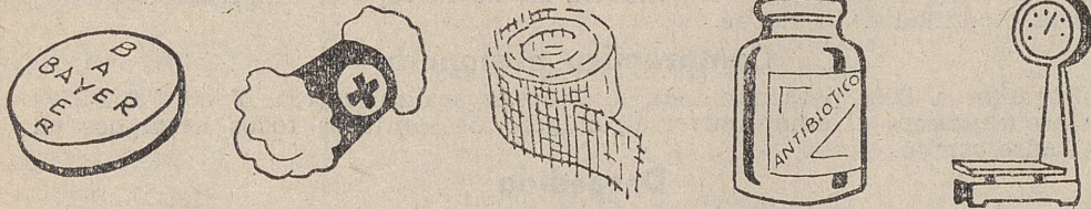
ANTIBIOTIQUES «antibiotik»
