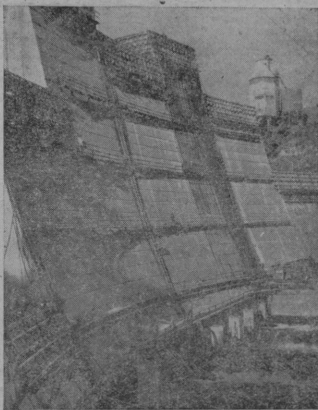
La presa Clark de la isla de Tasmania es la de mayor altura de Australia. El muro tiene más de 60 metros de altura y permite embalsar casi 300 millones de metros cúbicos de agua. Se podrán obtener, luego de instalada toda la maquinaria, 155.000 caballos de vapor.
