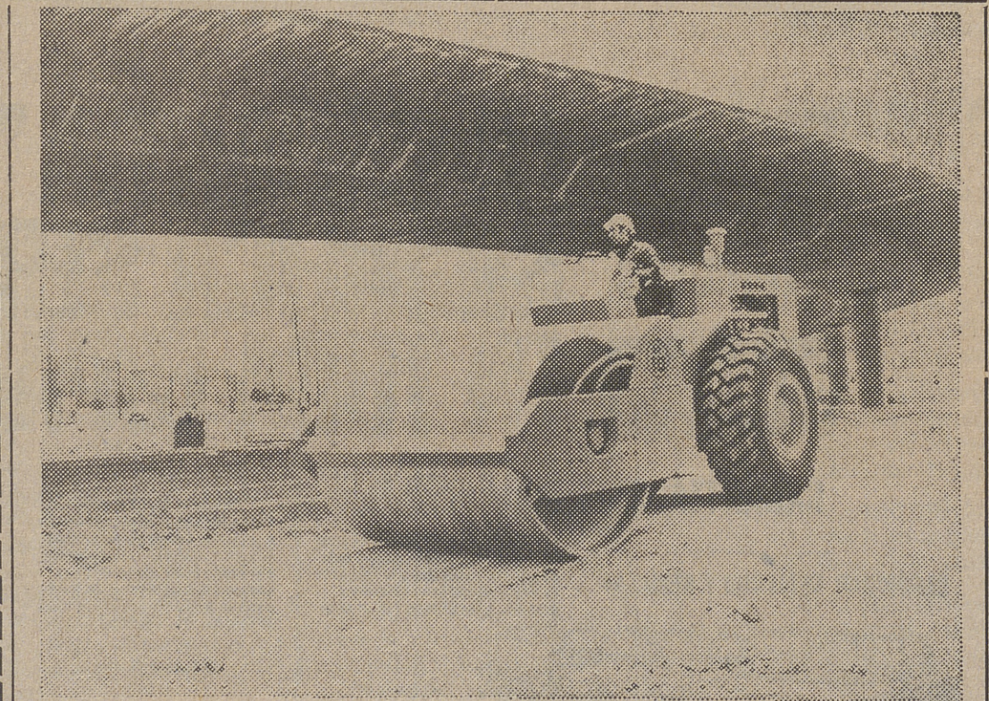
NOVEDAD DE MOTOR IBERICA, S. A.: Rodillo autopropulsado EBRO con motor Perkins de 6 cilindros y 90 HP, a 2.600 r.p.m., y peso en orden de marcha de 10 toneladas. Con transmisión hidrostática a las dos ruedas motrices. Seis velocidades, máxima de 25 kilómetros/hora y mínima en orden de trabajo de 0 a 2,5 Km./h. El caudal de la misma es de caudal fijo Sauer Solm, con válvulas limitadoras de presión taradas a 350 Kg./cm 2 . La presión normal es de 70 Kg./cm 2 . Dirección articulada y de accionamiento totalmente hidráulico, lo que facilita la maniobrabilidad del compactador. Diámetro de rodillo 1.500 milímetros. Con chapa de 25 mm. de espesor. Ancho de trabajo 2 m. Distancia entre ejes, 2,80 m. Longitud total, 5,15 m. Una buena noticia para los clientes y usuarios del sector de compactación.
