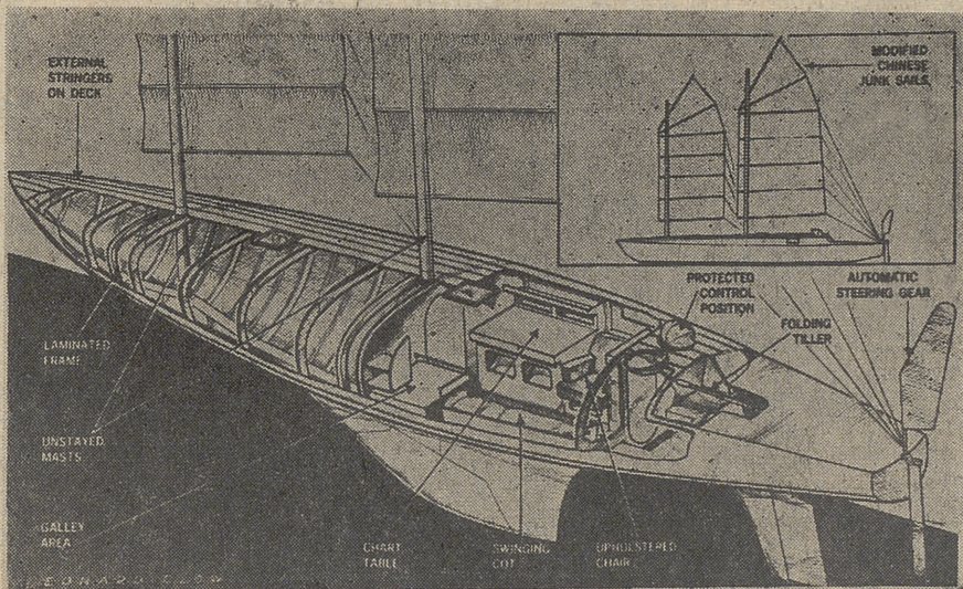
Diseño del «Blazer II» con el que Bill King se propone dar la vuelta al mundo.—FOTO EUROPA PRESS
