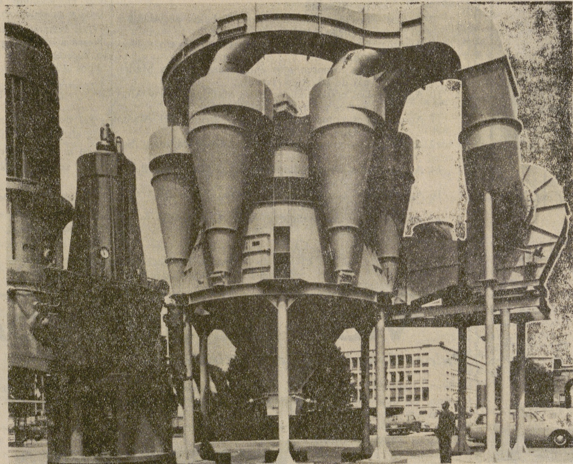
A un gigantesco pulpo de una película utópica se asemeja este monstruo de acero. Se trata en realidad de una máquina para el secado de cemento la que estaba exhibida en la "Achema 67", la feria y exposición de aparatos químicos celebrada en Francfort del Meno. Par-
