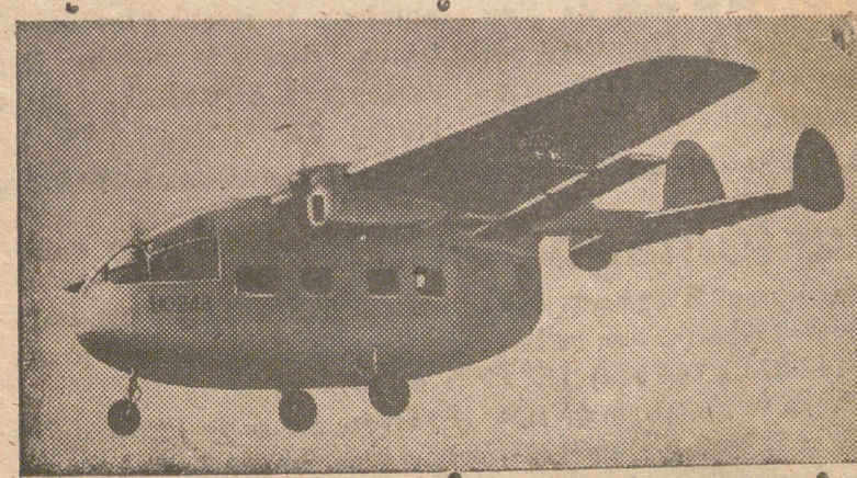
Avión «Aerovan» que lo mismo puede emplearse como ambulancia; para pasajeros y otros usos que para cargar en su amplio fuselaje un coche de cuatro plazas, dejando además sitio suficiente para los pasajeros.
