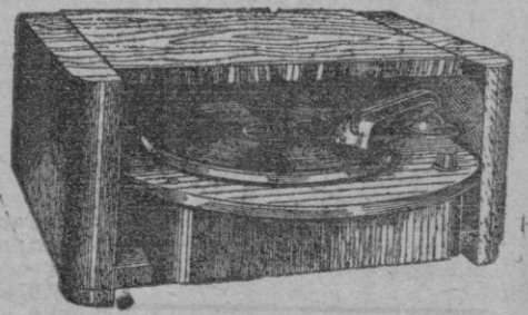
Tocadiscos marca F.E.A.R.E. Pick up de cristal, cuarzo; puesta en marcha y paro automáticos; adaptables a cualquier aparato con solo conectar un enchufe. Sistema de plataforma patentado. Precio v. p. 855 pts. (i. i.) Tocadiscos VERTOR; similares características anterior. Precio v. p. 725 pesetas (i. i.)
