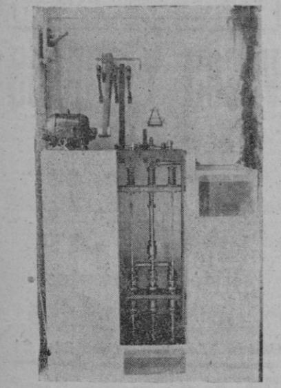
El modelo de bomba para sacar agua expuesto en la Feria por la Fundición Mallorquina
