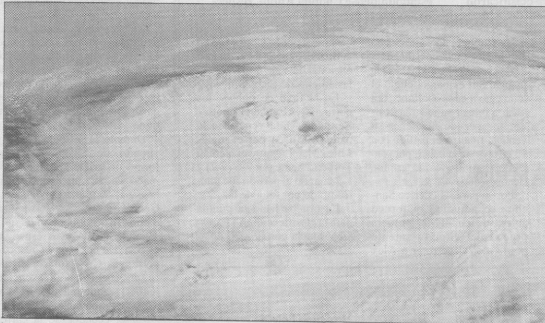
Imagen de un huracán tomada desde el transbordador espacial Discovery.
