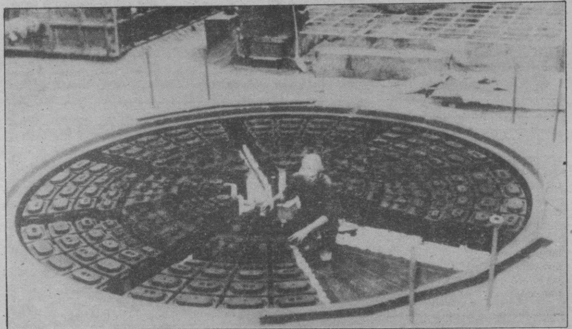
En la fotografía se capta la construcción de una gran pieza de hierro colado en los talleres de fundición del consorcio industrial Mannesmann Demag AG, de Duisburgo (República Federal de Alemania).
