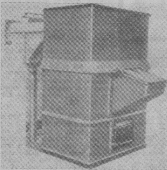
Incinerador para destruir basuras y desperdicios en granjas avícolas, mataderos, mercados, etc.
