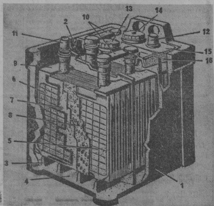
1, Recipiente. 2, Tabique que separa los vasos. 3, Nervios para apoyo de las placas. 4, Espacio para sedimentos. 5, Placa positiva. 6, Placa negativa. 7, Separador en contacto con la placa negativa. 8, Separador en contacto con la placa positiva. 9, Puente de unión de las placas negativas. 10, Puente de unión entre dos vasos. 11, Borne negativo. 12, Borne positivo. 13, Tapón del vaso. 14, Repiradero del tapón. 15, Cubierta de un vaso. 16, Material de relleno.
