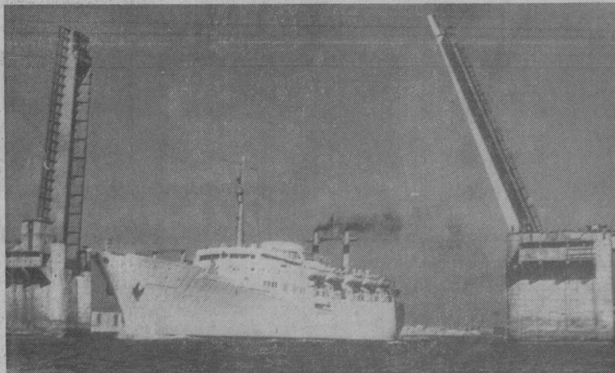
De Dortmund (Alemania Occidental) nos llega esta foto del mayor puente basculante doble del mundo que, esta vez, se encuentra en España. Es el construido sobre la bahía de Cádiz, levantado en cooperación con una empresa española por una planta siderúrgica alemana de Dortmund. En sólo tres minutos se abren los tramos-báscula de sesenta y ocho metros de largo para dejar pasar buques por el canalizo de noventa de ancho. Cerrado el puente pueden pasar bajo el buques de hasta veintidós metros de altura. (Foto DaD)
