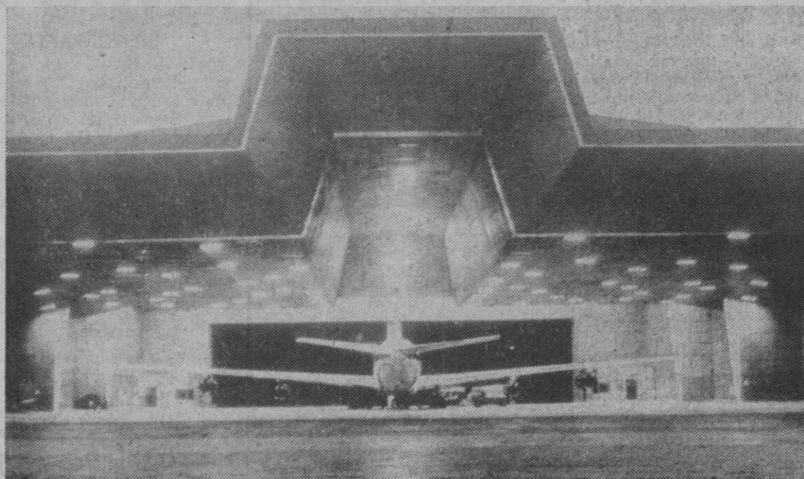
Hamburgo.—Este hangar antiacústico es la obra más singular del aeródromo de Hamburgo. Es única en la República Federal de Alemania, quizás hasta en el mundo. Fue construida por físicos e ingenieros y costó más de nueve millones de marcos. Tiene por sentido y objetivo cuidar los nervios de los vecinos del terreno del aeródromo. Incluso los grupos de aviones de reacción más grandes pueden marchar aquí durante horas enteras con alto número de revoluciones sin que casi se perciba ningún sonido fuera. Con todo eso el hangar antiacústico hamburgués no tiene ninguna puerta. Su abertura se encuentra en dirección de la región menos poblada. Las paredes y los ríncones están revestidos de material fonoabsorbente y las paredes están escalonadas así que el ruido no absorbido es repellido hacia el interior del hangar.—(Foto DaD)
