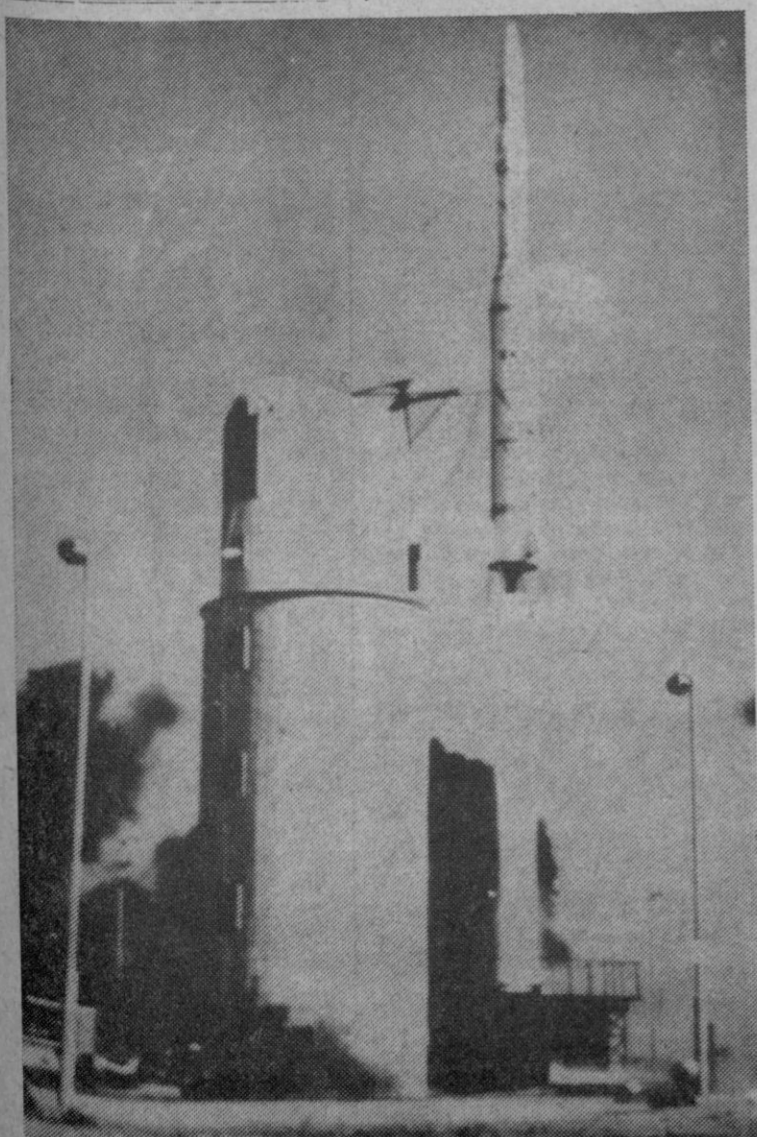
Hammaguir.—El satélite francés «Diadème» fue lanzado en la base de Hammaguir en el Sahara argelino. Momento en que se despara el cohete «Diamant» portador del «Diadème»
