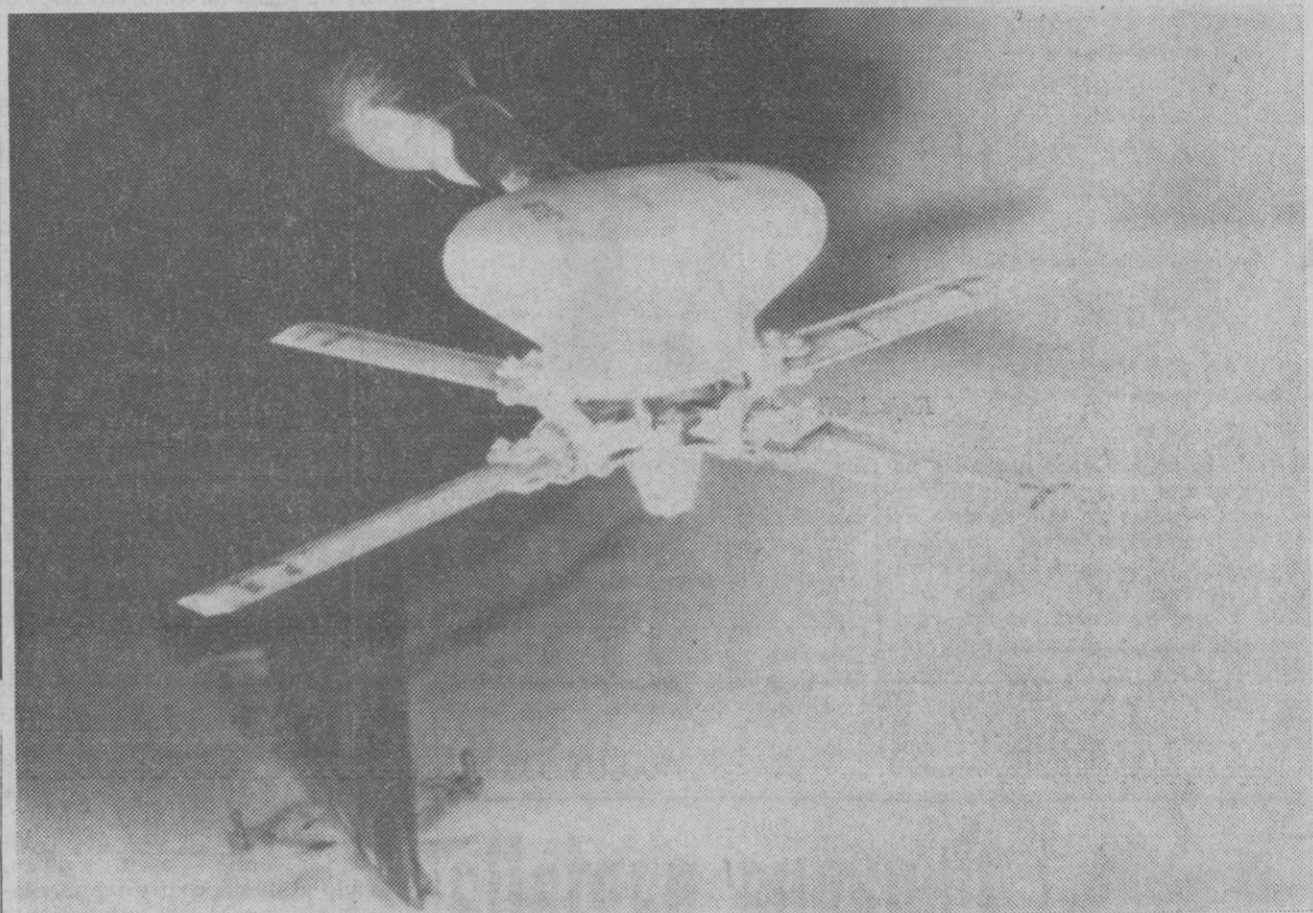
Centro de Investigación Ames, Mountain View (California).—Maqueta de un vehículo para regresar del espacio a la atmósfera terrestre, de aplicación para los vuelos espaciales. Los rotors de que va dotado se despliegan parcialmente hasta alcanzar una altura prudente y, a continuación se despliegan como en esta foto para aterrizar en el suelo. La N. A. S. A. lo está proyectando para velocidades superiores a las dos mil trescientas millas por hora. (Foto Europa Press)
