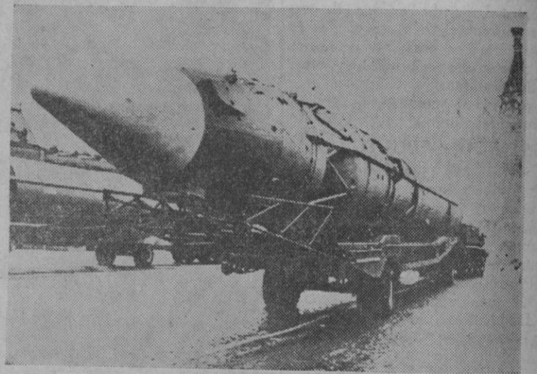
Dos de los misiles de tres fases que participaron en el desfile del aniversario de la revolución de octubre en la Plaza Roja de Moscú. Según los soviéticos, estos misiles pueden ser puestos en órbita alrededor de la tierra para lanzarse con su carga atómica sobre cualquier objetivo.—(Foto Fiel)
