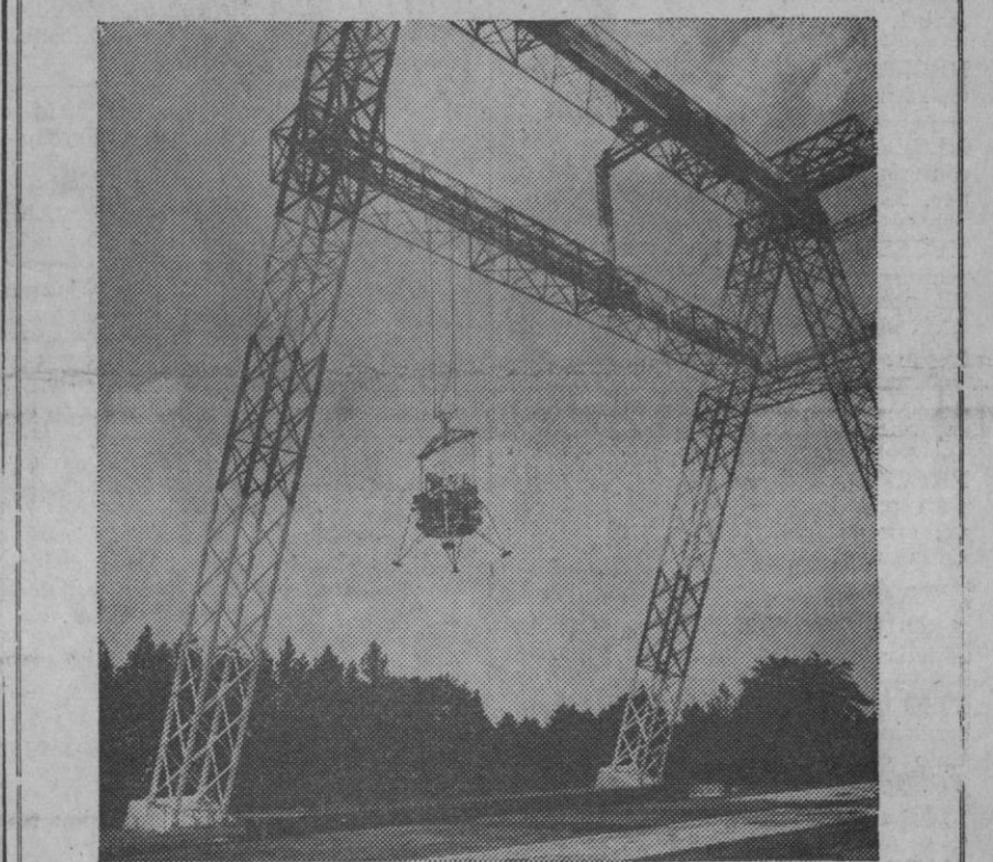
Los métodos para el descenso del vehículo tripulado Apolo en la superficie de la Luna están siendo ensayados y probados con este enorme aparato en el Centro Langley de Investigaciones, de Virginia. El vehículo se hace maniobrar por medio de breves impulsos producidos con un pequeño cohete y el sistema de armazón y cables simula la fuerza de gravedad lunar que es solamente una sexta parte de la terrestre. El aparato experimental tiene más de 75 metros de alto por 120 de largo
