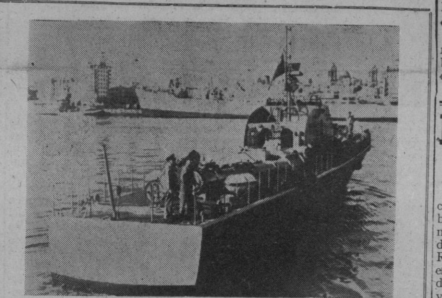
Cádiz.—Se celebró en esta ciudad la entrega de la lancha rápida "Guacolda" a la Marina chilena. La embarcación, construida en la factoría gaditana de la Empresa Nacional Bazán, es la primera de una serie de cuatro concertada con la Marina de aquel país andino. En la foto, la "Guacolda" en el puerto de Cádiz.
