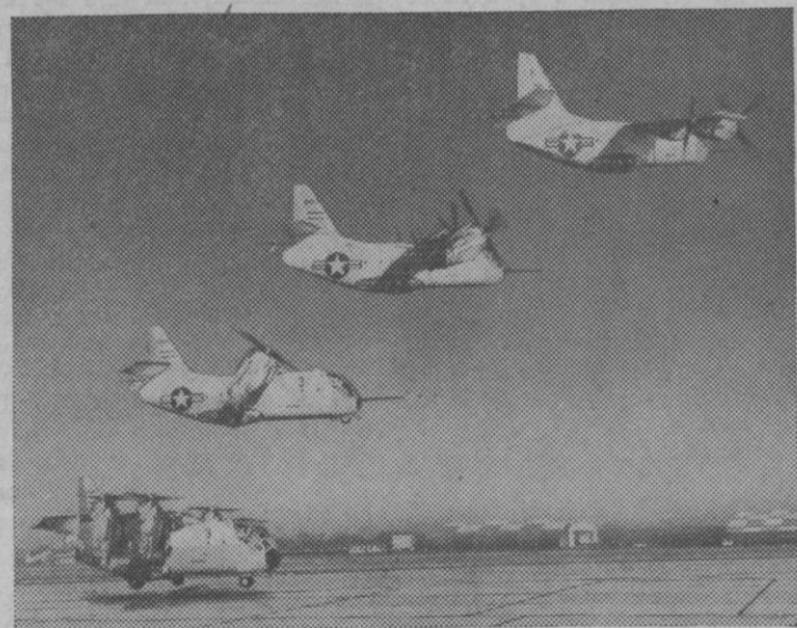
La foto compuesta ilustra el despegue y transición al vuelo frontal del transporte aéreo XC-142A. El aparato despega verticalmente como un helicóptero con las alas en posición vertical. A medida que el avión gana altura las alas van bajando para el vuelo a alta velocidad. El XC-142A está en periodo de pruebas en la Ling-Tenco-Vought, Dallas (Texas), y está destinado a las fuerzas armadas de los Estados Unidos
