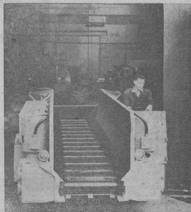
Nuevo modelo de vagoneta lanzadera, de las que se emplean extensamente en la minería metalífera en gran escala y en la explotación hullera de todo el mundo, con una capacidad de quince toneladas. Este vehículo incorpora dirección y frenaje ayudados a potencia, tiene una conductora más poderosa y, entre otros rasgos, reduce la fatiga del conductor y permite mayor capacidad de trabajo
