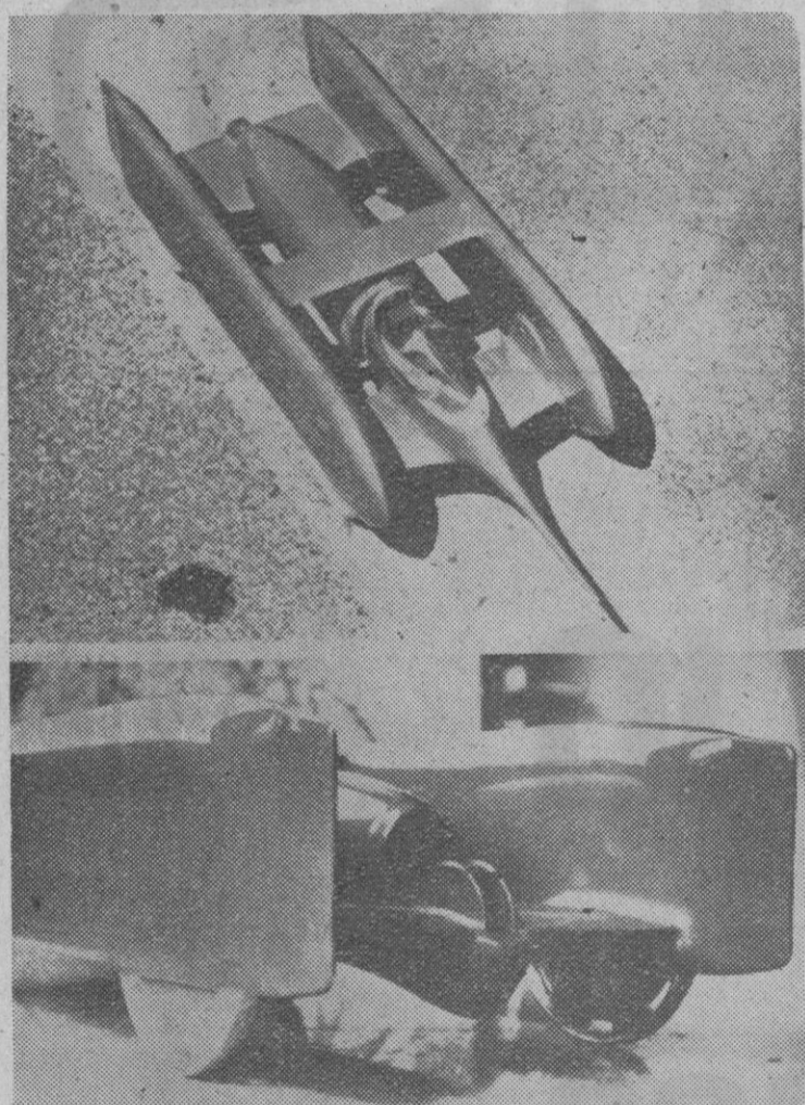
Este sensacional vehículo ha sido diseñado por el alemán Leopold Schmid, de Stuttgart, y él mismo piensa terminar la construcción en 1965. Con el automóvil tratará de alcanzar los mil kilómetros por hora, superando así el récord mundial conseguido en 1947 por el americano John Cobb (634,4 kilómetros hora). El único instrumento que tendrá el conductor en la cabina será un cuentakilómetros. En la foto de arriba, el diseño de Schmid, y en la de abajo, el eje posterior del mismo.—(Foto Fiel.)
