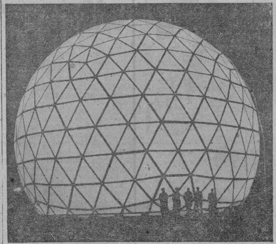
Esta gigantesca cúpula de plástico, que mide veintidós metros de diámetro y unos quince de altura, ha sido diseñada para proteger equipo de radar y puede resistir vientos huracanados y temperaturas bajo cero. Consta de trescientas secciones grandes, empennadas, y se dice que es la mayor estructura de plástico reforzado hecha hasta ahora en Europa
