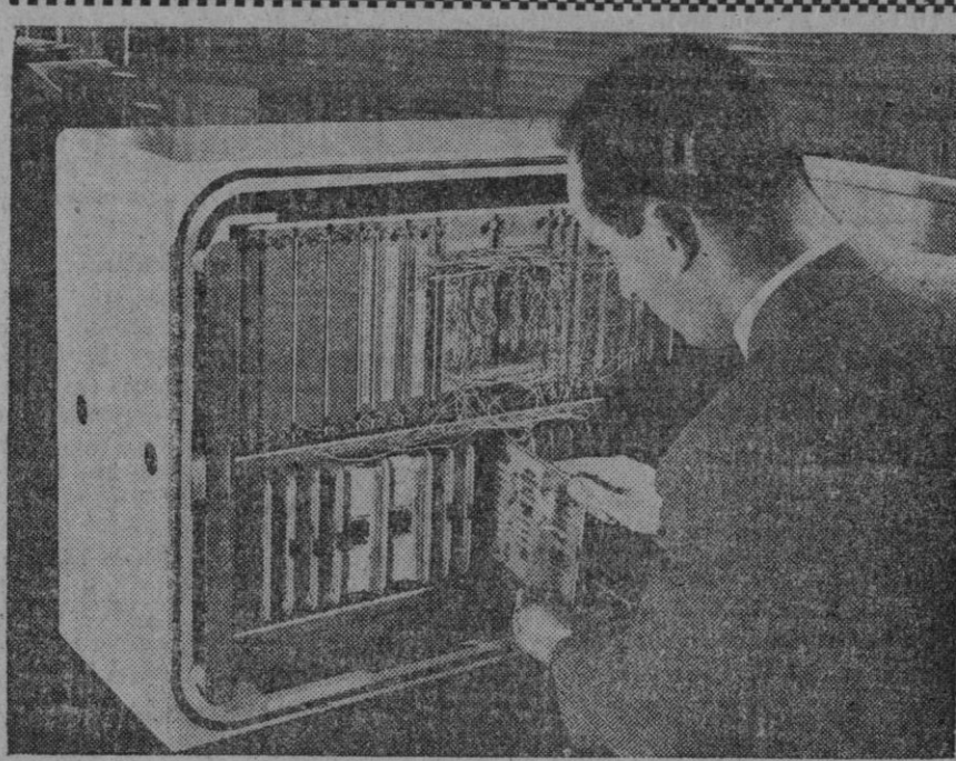
Esta nueva, y notablemente barata, calculadora análoga, diseñada especialmente para las industrias de transformación, se exhibirá en la Exposición Interkama, que se celebrará en Dusseldorf en este mes. En esta fotografía, el operador inserta en la calculadora una tarjeta con circuito estampado. Mediante el empleo de circuitos estampados se consigue usar el mínimo número de elementos para resolver un determinado problema. La calculadora, llamada Anatrol, puede vigilar y controlar automáticamente una amplia variedad de procesos de fabricación. La producción de petróleo, substancias químicas derivadas de él y alimentos líquidos son aplicaciones para las cuales es idealmente adecuada.
