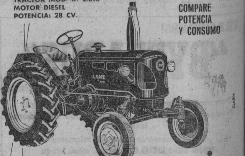
TRACTOR MOD. D. 2.816 MOTOR DIESEL POTENCIA: 28 CV.
