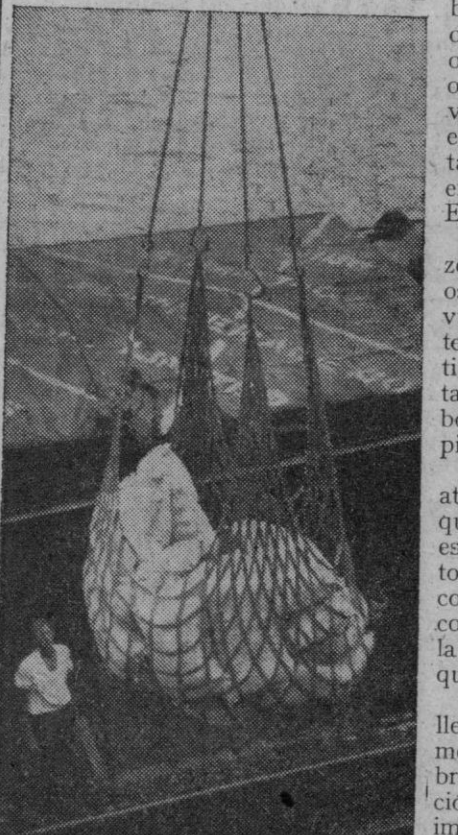
Descarga de harina, con un nuevo tipo de red fabricada de tejido oblongo de nylon. Esta red, liviana, flexible y fácil de manejar aunque esté mojada, es muy fuerte y de gran duración. La red que se ve en la fotografía mide 1,3 metros cuadrados y pesa solamente 11,25 kilogramos, pero ha levantado durante las pruebas pesos de dos toneladas con completa seguridad. El nylon es mucho más resistente que el material empleado ahora generalmente en la fabricación de redes, permanece enteramente flexible en toda clase de condiciones y no se pone rígido ni duro al mojarse. Además, es inmune a la podredumbre y al ataque del agua del mar y posee una notable resistencia a la abrasión. Otra de sus ventajas es la facilidad de limpieza.
