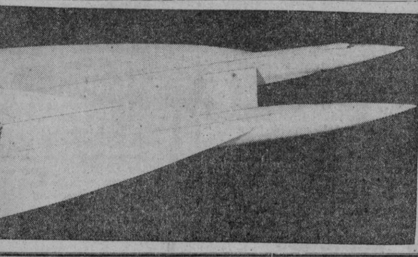
Modelo de uno de los posibles proyectos de un avión dotado de una velocidad de tres mil doscientos kilómetros por hora, para ciento treinta pasajeros, diseñado recientemente por el doctor R. Jamison, jefe del departamento de estrato-reactores de la firma británica Bristol Siddeley Engines Ltd. El avión estaría propulsado por estrato-reactores y turbo-reactores
