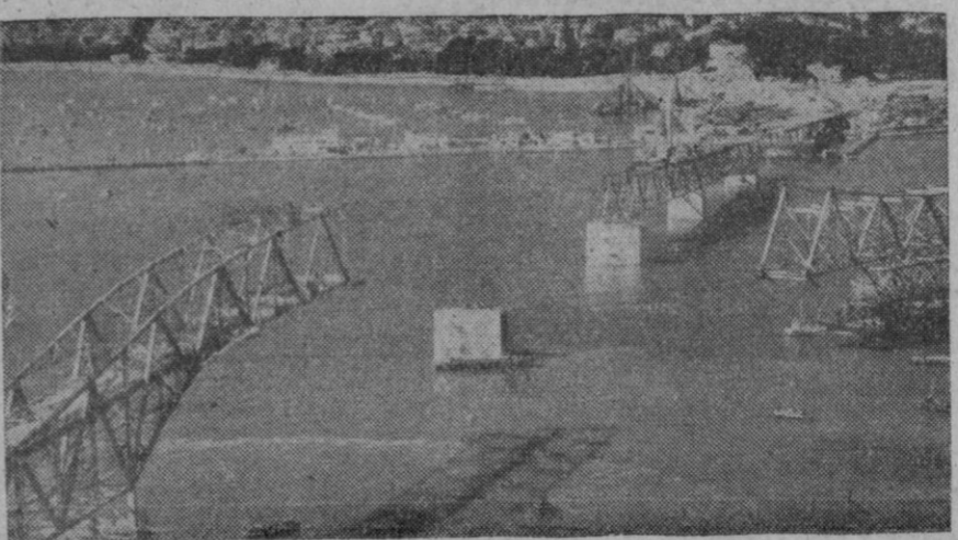
Se muestra en esta fotografía uno de los tramos principales del nuevo puente en Auckland, que ahora se construye en Nueva Zelanda, en el momento en que flota en posición durante la marea alta. Con sólo el referido tramo, que pesa 1.200 toneladas, y tiene una longitud de 183 metros, dicho puente será el más largo que se ha completado, durante los últimos veinte años, en el Hemisferio Sur. El nuevo puente servirá para enlazar la ciudad de Auckland con el burgo de Northcote. Los trabajos se iniciaron a principios de 1955, y la obra completa se espera que termine en Mayo de 1959
