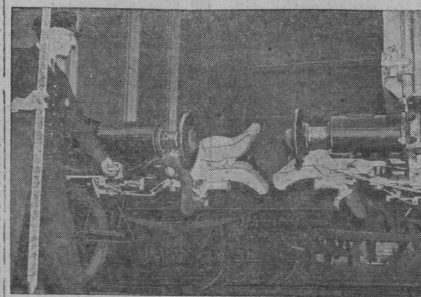
En la exposición celebrada recientemente con el nombre de «Transports de carga» en Battersea (Londres), se exhibió este enganchado automático de vagones que constituye una valiosa aportación al programa de modernización de los ferrocarriles, pues aumenta considerablemente la eficiencia y la rapidez de las maniobras, reduciendo al mismo tiempo el peligro de accidentes. Es de operación completamente automática, incorpora conexiones simultáneas del tubo de freno al vacío y se puede emplear con todos los vagones que se utilizan actualmente
