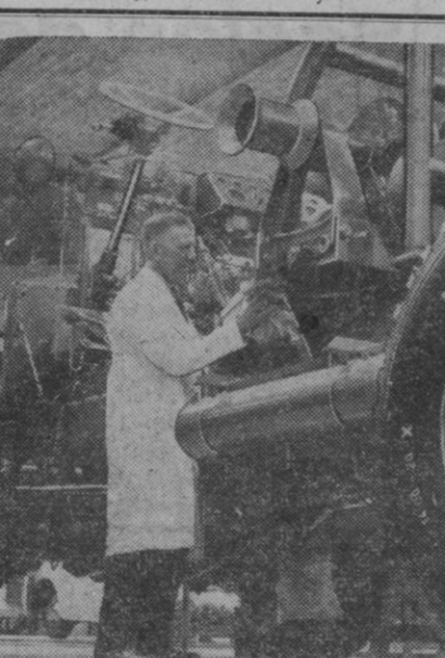
Diseñado para operaciones en el desierto o en cualquier terreno accidentado, como, por ejemplo, para remolcar equipo de perforación y prospección petrolera, este nuevo tractor, el «Super Constructor», pesa, con remolque, setenta y cinco toneladas. Está propulsado por un motor diesel de doscientos treinta caballos al freno, que impulsa al vehículo y su carga sobre terrenos arenosos y fangosos, empleando una caja de cambios automática con ocho velocidades y transmisión a las seis ruedas. Está provisto también de tornos que pueden desarrollar un esfuerzo tractor de veintisiete toneladas.
