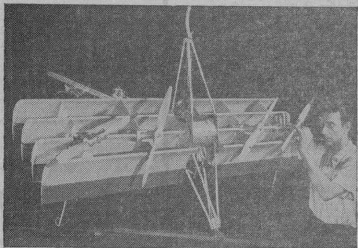
Aunque el aparato ofrezca un aspecto raro, se trata de un avión experimental que puede volar verticalmente. Ideado para realizar el trabajo de un helicóptero, tendrá una velocidad mucho mayor. Las cuatro alas desvían hacia abajo la corriente de aire de la hélice para imprimir el movimiento vertical hacia arriba. Una vez en el aire se cambia el ángulo de las alas y ya está logrado el vuelo corriente
