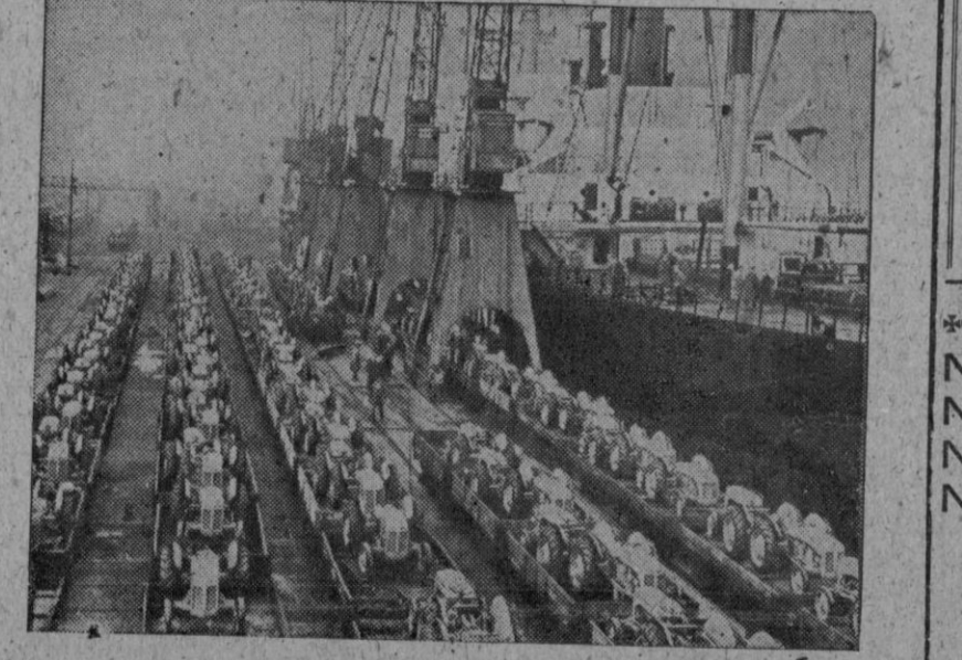
Embarque en un puerto inglés, de tractores "Ferguson", con destino a los Estados Unidos. El barco no llevaba otra carga y se tardaron siete horas en embarcar 633 vehículos
